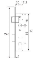
FZD-07HL Material: Aluminum alloy
