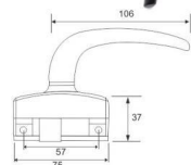
FZD-13HU (Oblique) Material: Aluminum alloy semi zinc aluminum
