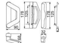
FZD-07HL Material: Aluminum alloy
