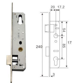
FZD-07HL Material: Aluminum alloy
