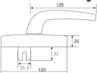
FZD-07HU Material: Aluminum alloy
