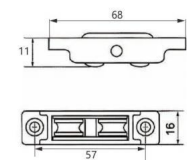
FZD-36R Material: Iron
